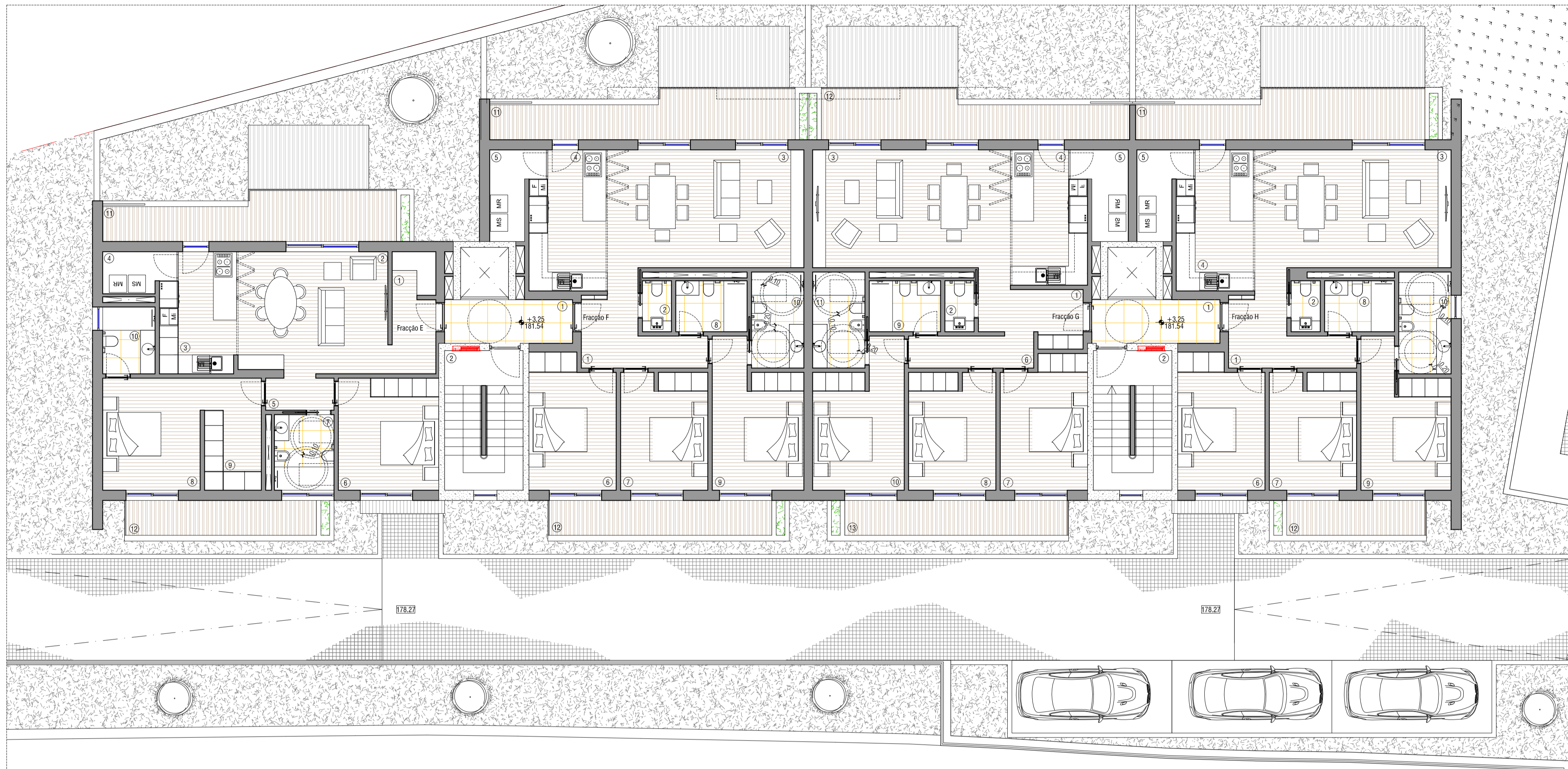
PLANTA DE PISO 2
