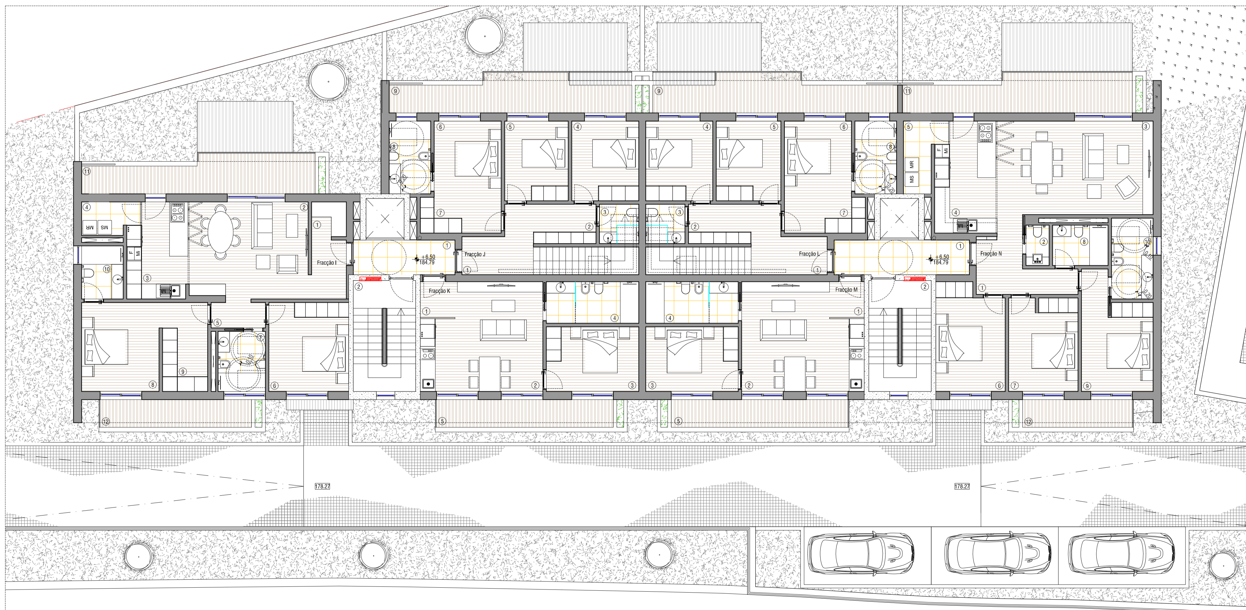
PLANTA DE PISO 3
